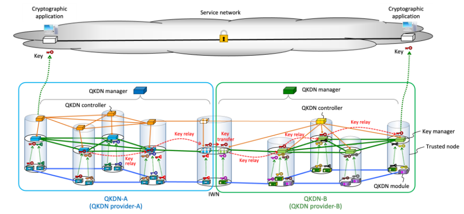
QKDNインタワーキング構成図
