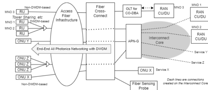
IOWN GFアーキテクチャによるアクセス網構成例
