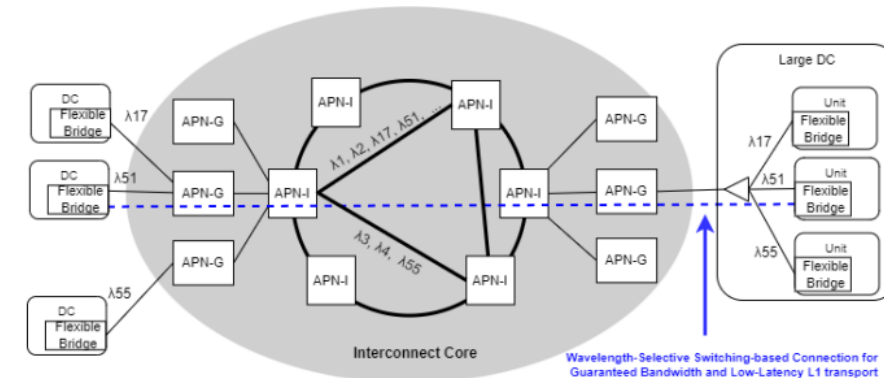
IOWN GFアーキテクチャによる基幹網構成例
