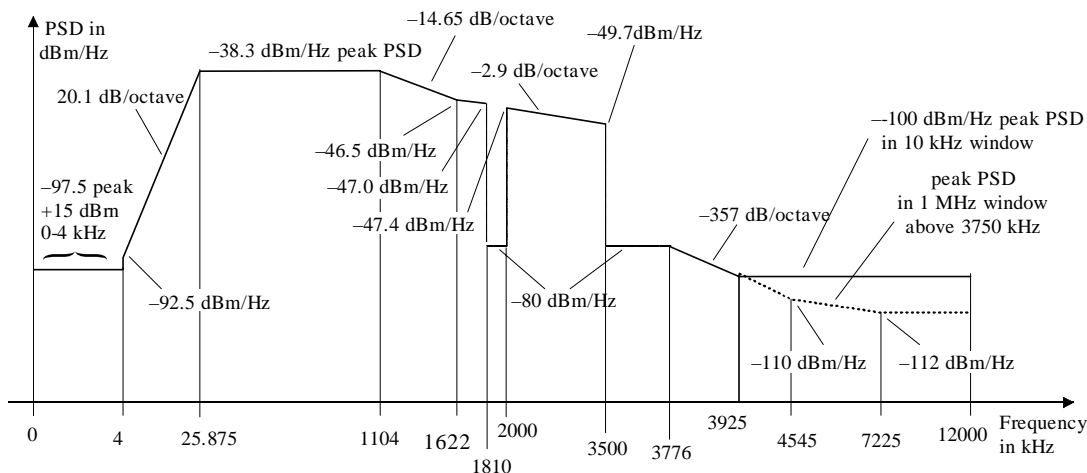
図 1 クアッドスペクトルオーバーラップマスクとピーク値に基づくプロット
