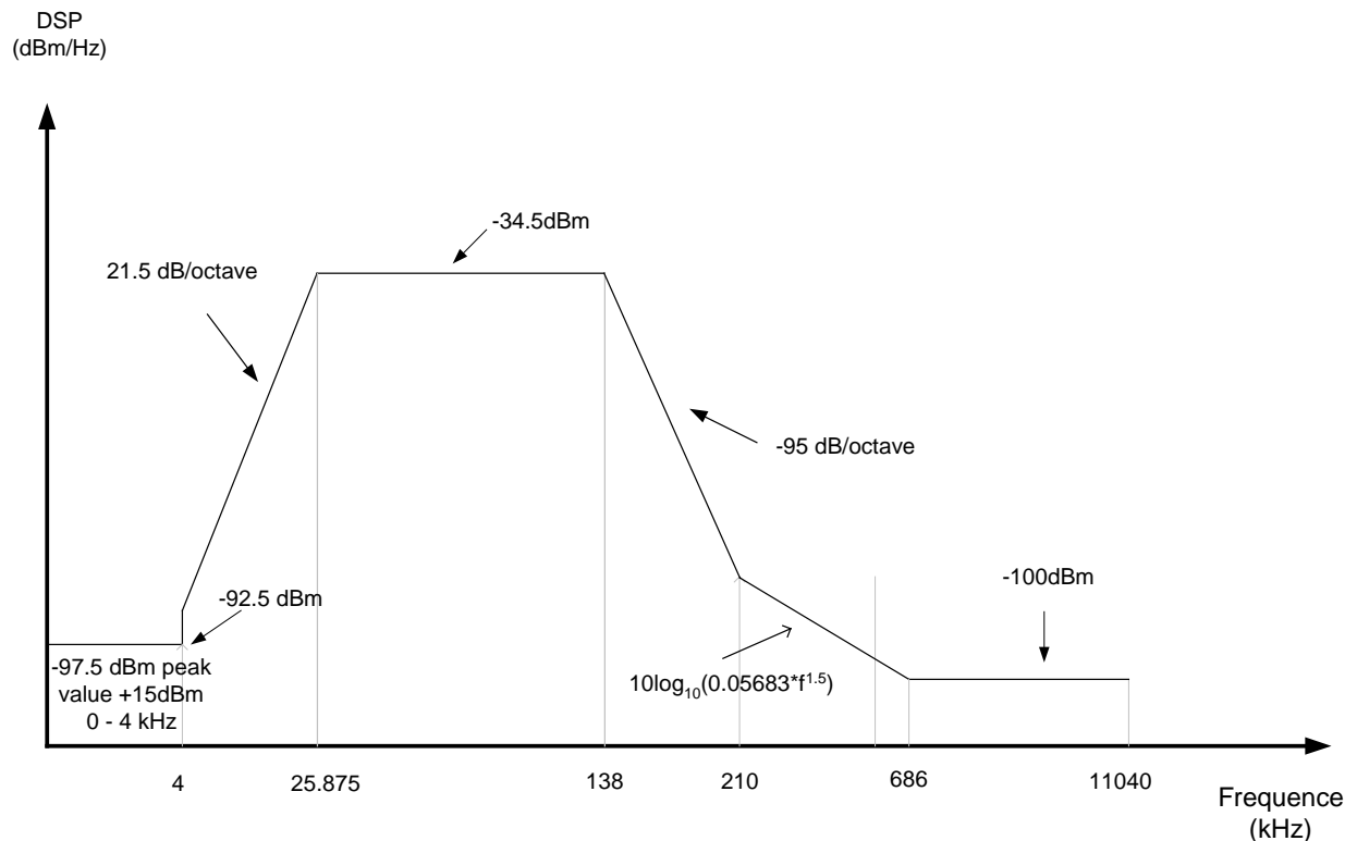
図 2 G.992.5 のアップストリームマスク図（尖頭値）
