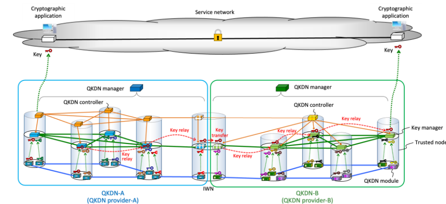
QKDNインタワーキング構成図
