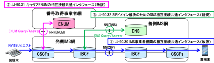
IMSネットワーク間の参照NNI
