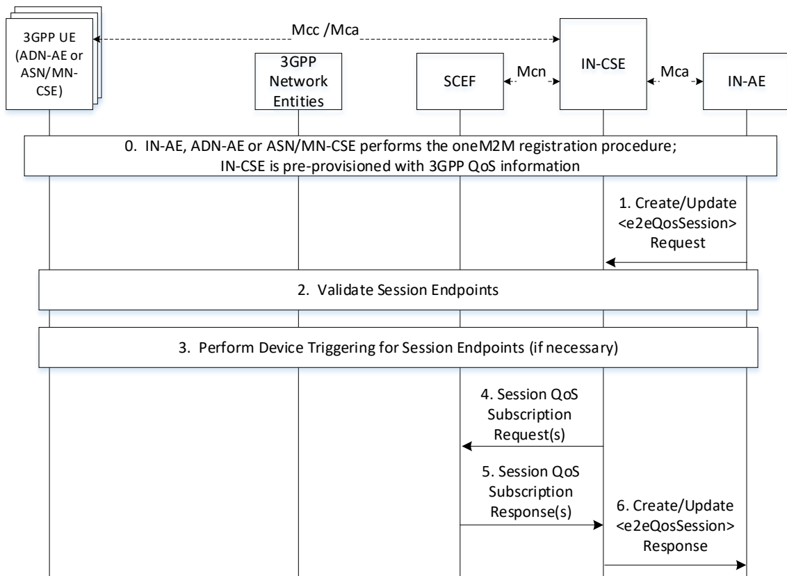
Figure 7.9.3.1-1: Create/Update E2E QoS procedure
