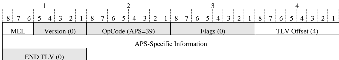
図 11-1/JT-G8031 – APS PDU フォーマット
