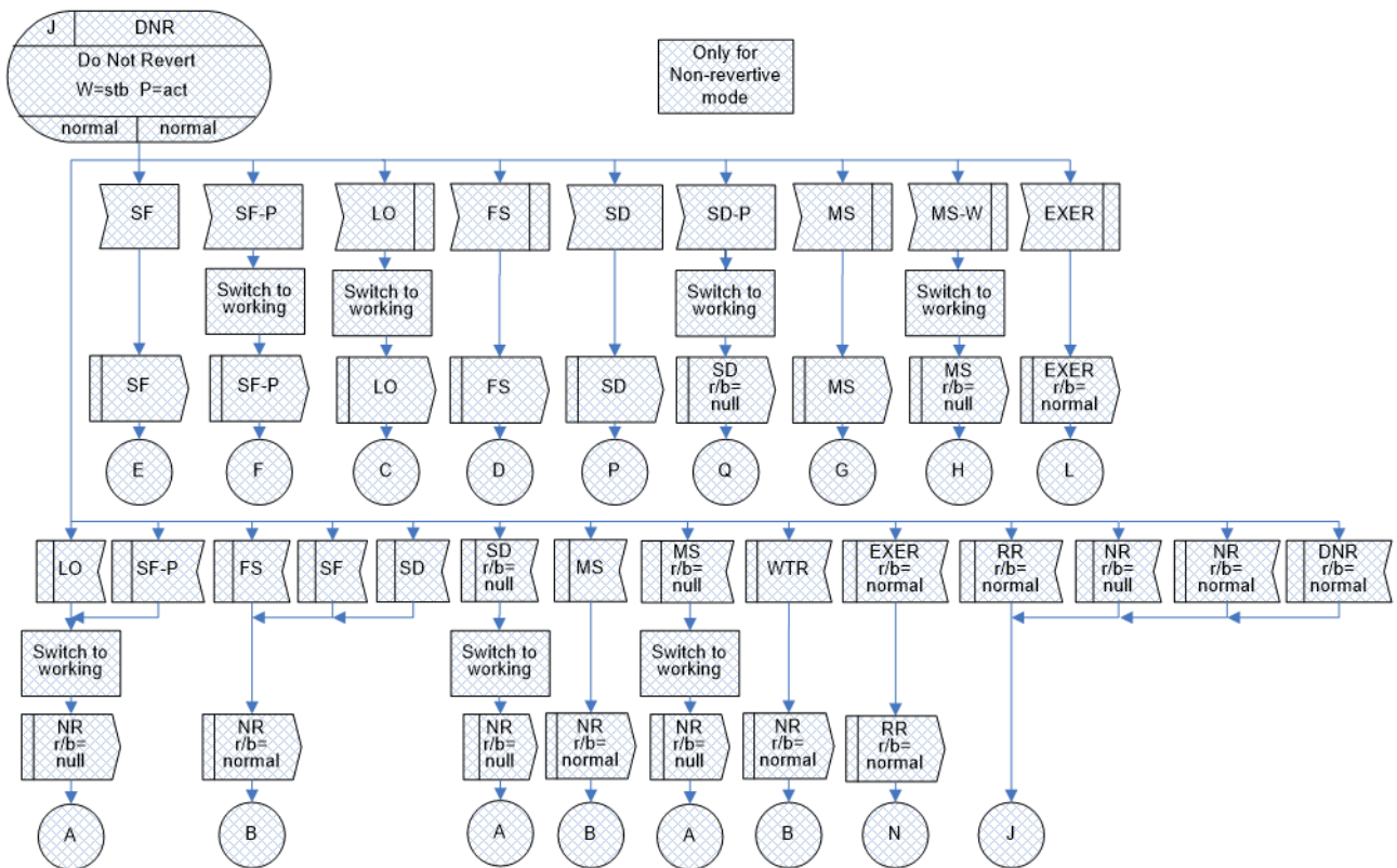
図 IV.10/JT-G8031 - 1:1双方向プロテクション切替におけるDNR(r/b=normal)状態
