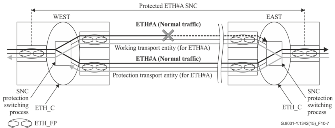
図10-7/ JT-G8031 - 1+1 片方向プロテクションアーキテクチャ -westからeast方向での運用系エンティティの信号故障（または信号劣化）状態
