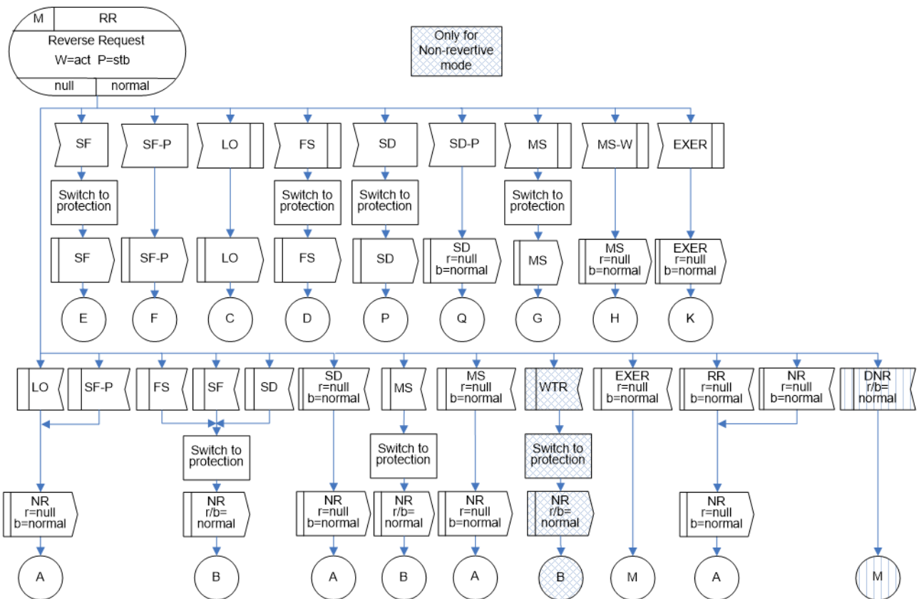
図 IV.29/JT-G8031 - 1+1双方向プロテクション切替におけるRR(r=null, b=normal)状態
