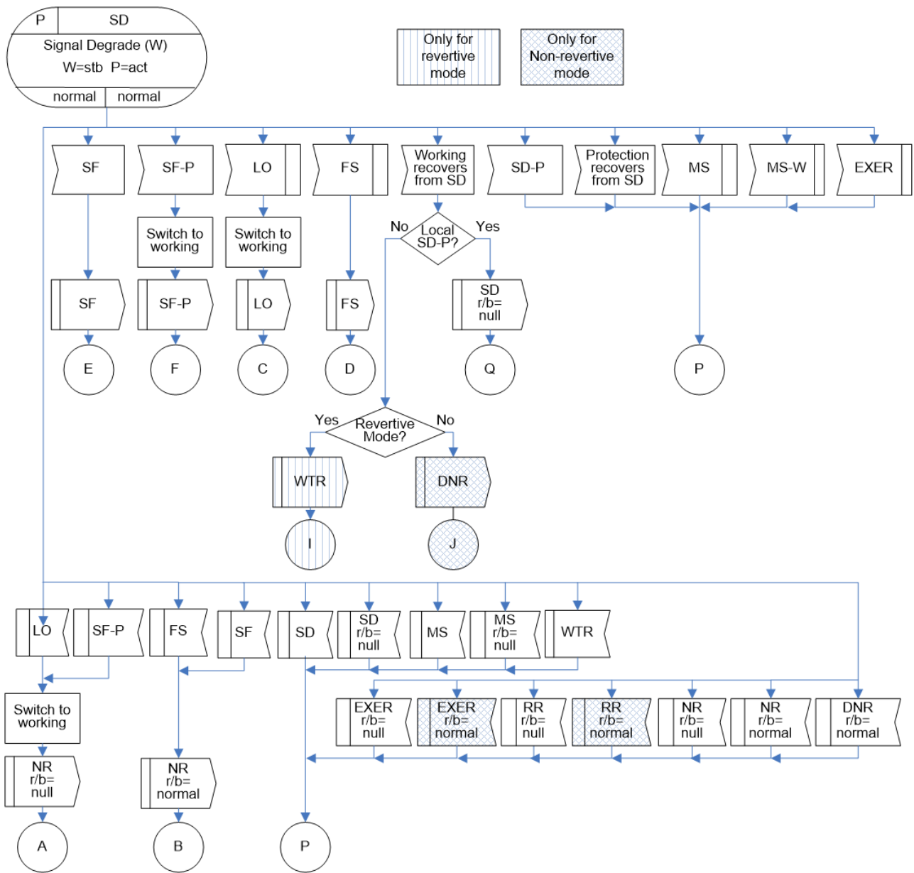
図 IV.15/JT-G8031 - 1:1双方向プロテクション切替におけるSD(r/b=normal)状態
