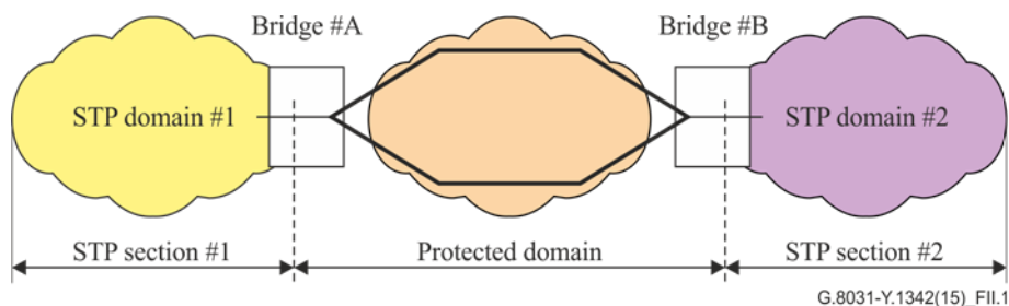
図 II.1/JT-G8031 -保護ドメインとSTPドメイン間で重複が無いケース
