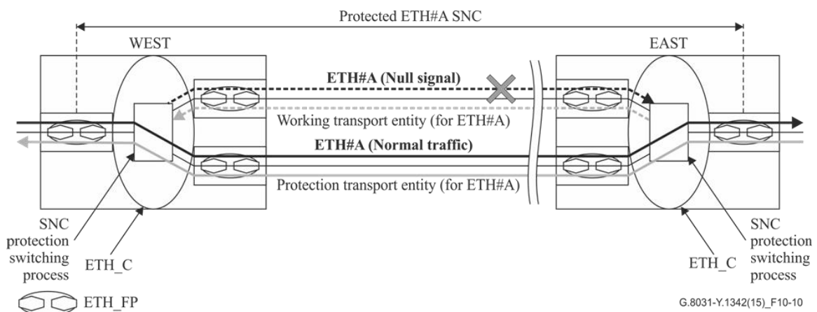
図 10-10/JT-G8031 - 1:1 プロテクションアーキテクチャ - (セレクトブリッジによる) - 運用系トランスポートエンティティの信号故障状態
