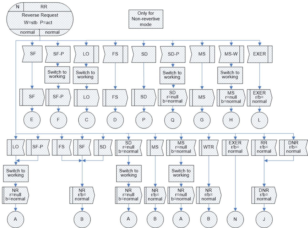
図 IV.30/JT-G8031 – 1+1双方向プロテクション切替におけるRR(r/b=normal)状態
