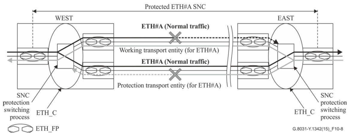
図10-8/ JT-G8031 - 1+1 片方向プロテクションアーキテクチャ -双方向での信号故障（または信号劣化）状態
