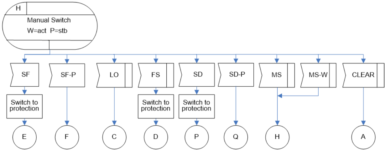
図 IV.39/JT-G8031 -1+1片方向プロテクション切替におけるMS(W=act / P=stb)状態
