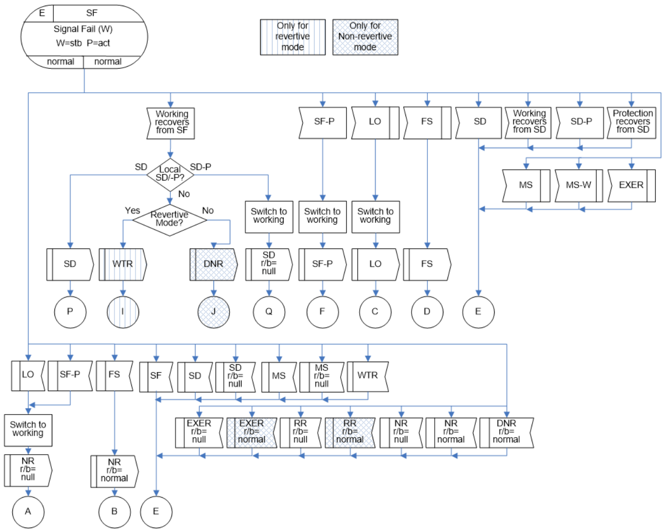
図 IV.5/JT-G8031 - 1:1双方向プロテクション切替におけるSF(r/b=normal)状態
