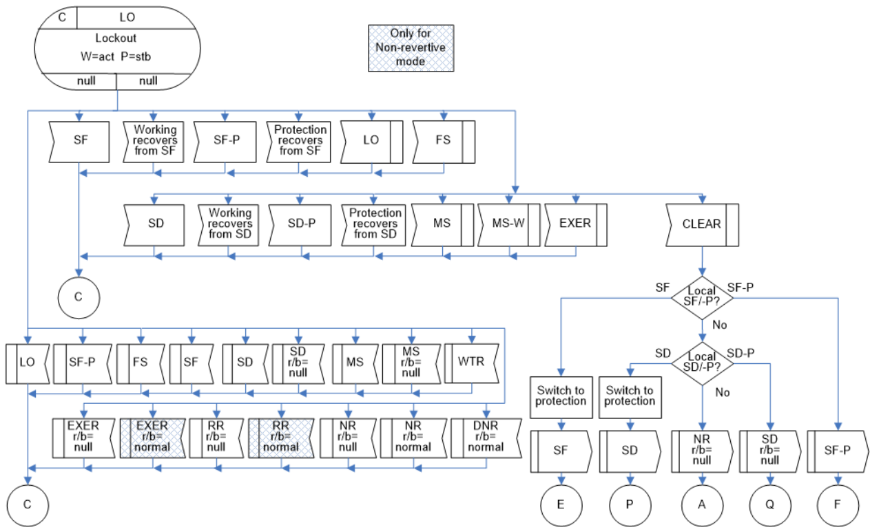
図 IV.3/JT-G8031 - 1:1双方向プロテクション切替におけるLO
