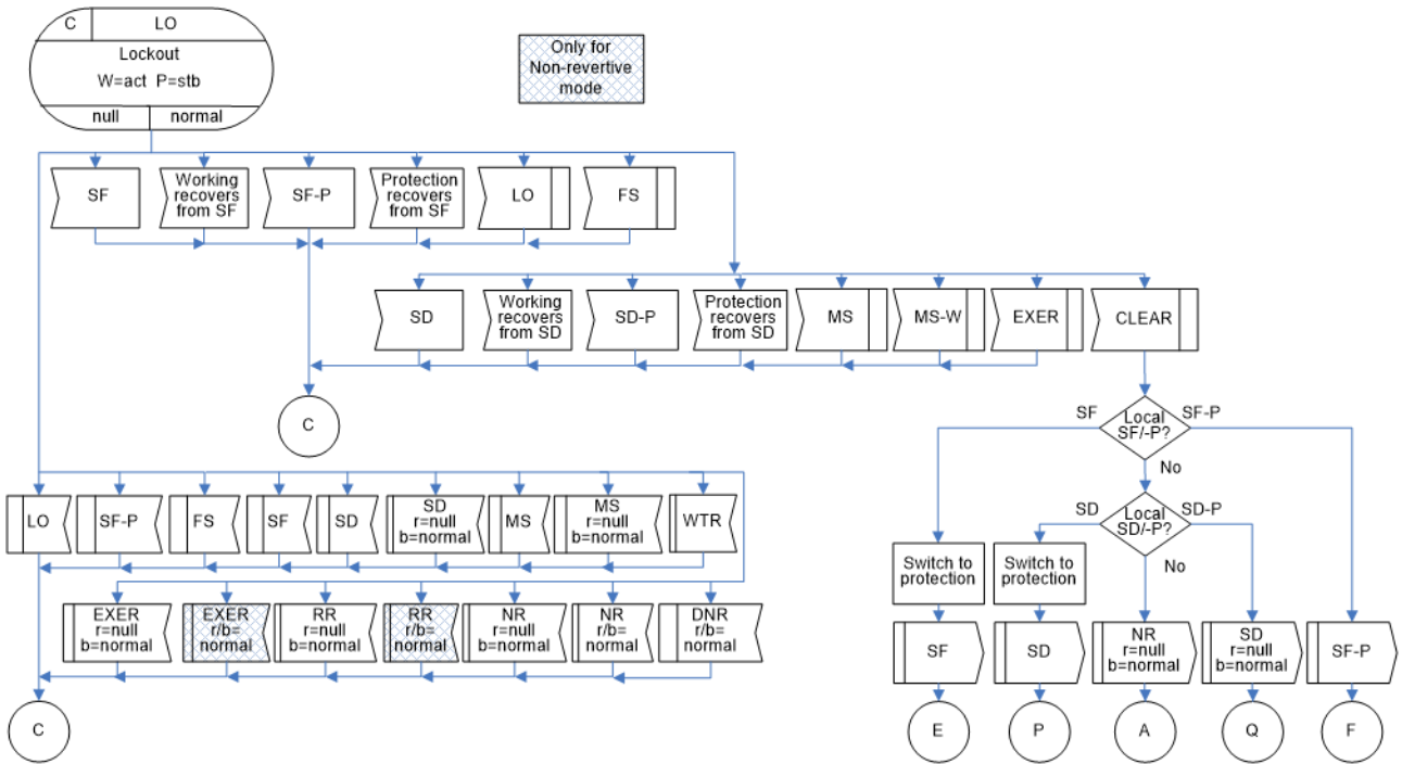
図 IV.19/JT-G8031 - 1+1双方向プロテクション切替におけるLO(r=null, b=normal)状態
