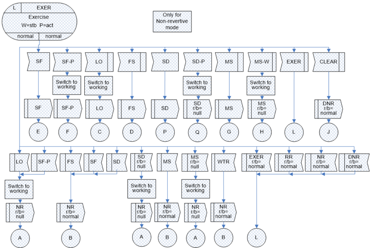
図 IV.12/JT-G8031 - 1:1双方向プロテクション切替におけるEXER(r/b=normal)状態
