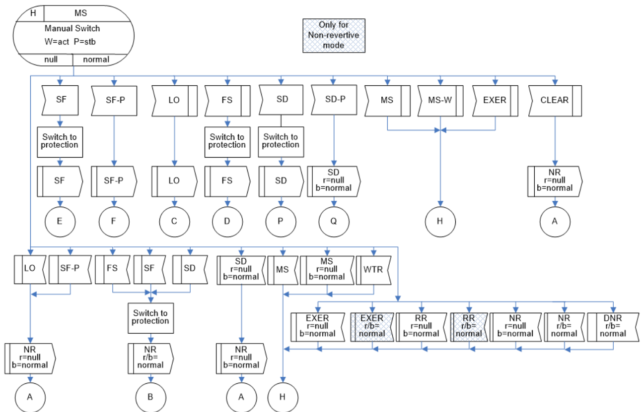
図 IV.24/JT-G8031 - 1+1双方向プロテクション切替におけるMS(r=null, b=normal)状態
