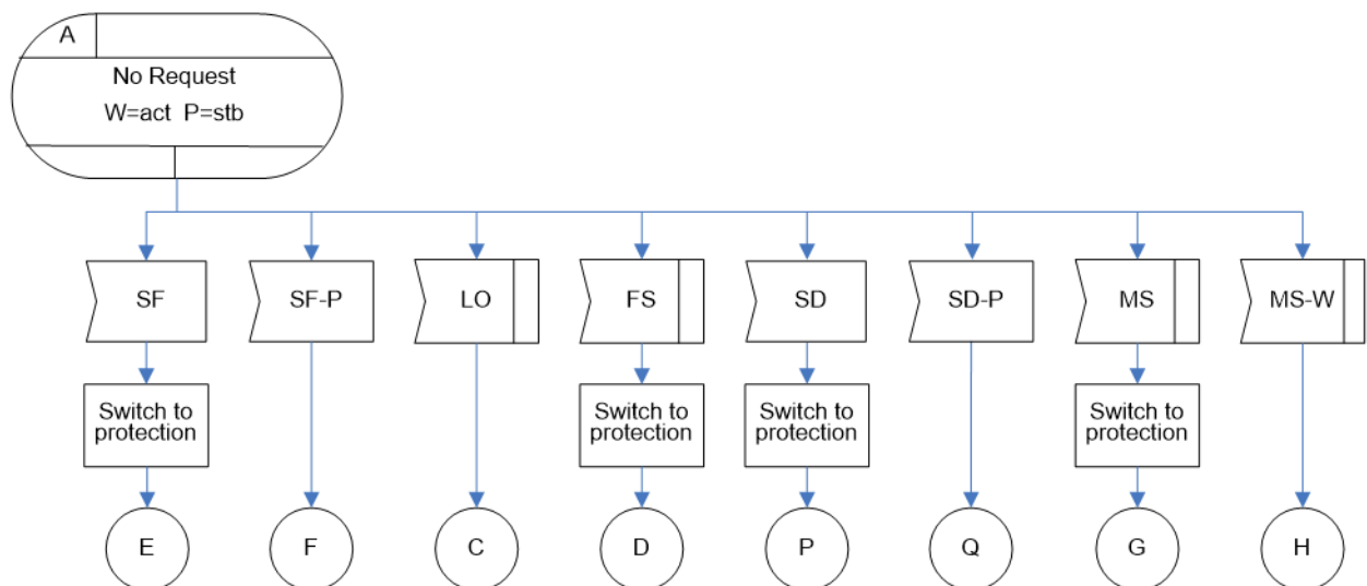
図 IV.33/JT-G8031 - 1+1片方向プロテクション切替におけるNR(W=act / P=stb)状態
