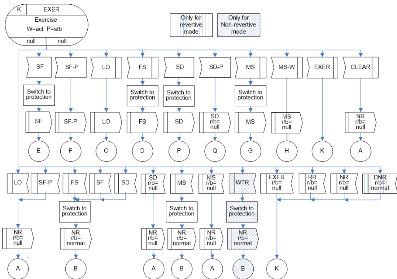
図 IV.11/JT-G8031 - 1:1双方向プロテクション切替におけるEXER(r/b=null)状態
