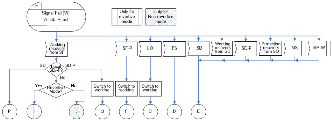
図 IV.36/JT-G8031 -1+1片方向プロテクション切替におけるSF(W=stb / P=act)状態
