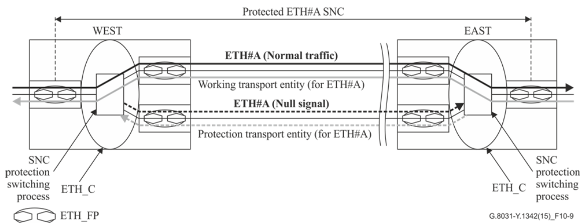
図 10-9/JT-G8031 -1:1 プロテクションアーキテクチャ
