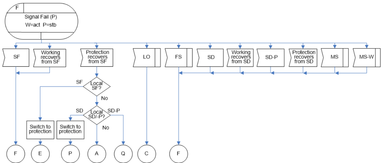
図 IV.37/JT-G8031 -1+1片方向プロテクション切替におけるSF-P(W=act / P=stb)状態
