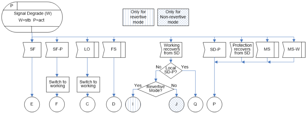
図 IV.42/JT-G8031 - 1+1片方向プロテクション切替におけるSD(W=stb / P=act)状態
