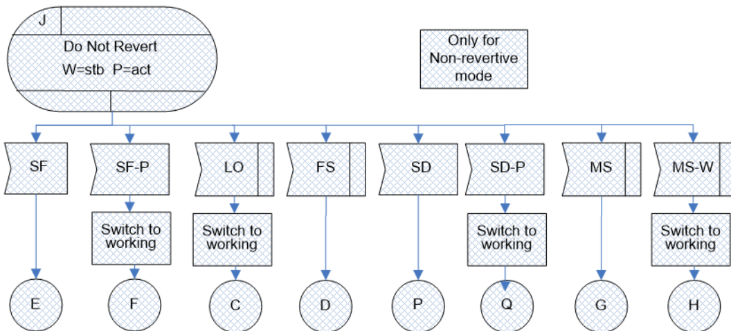
図 IV.41/JT-G8031 -1+1片方向プロテクション切替におけるDNR(W=stb / P=act)状態
