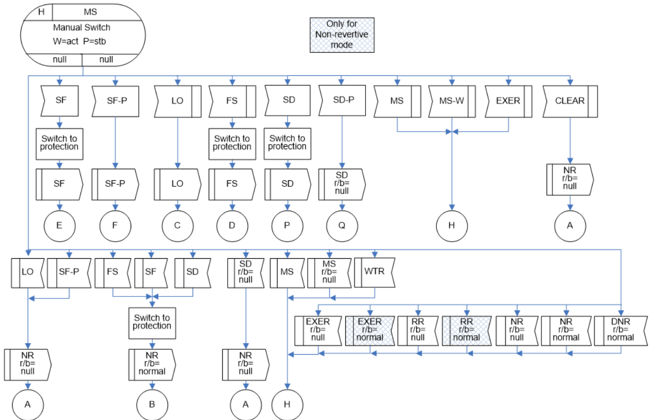
図 IV.8/JT-G8031 -1:1双方向プロテクション切替におけるMS(r/b=null)状態
