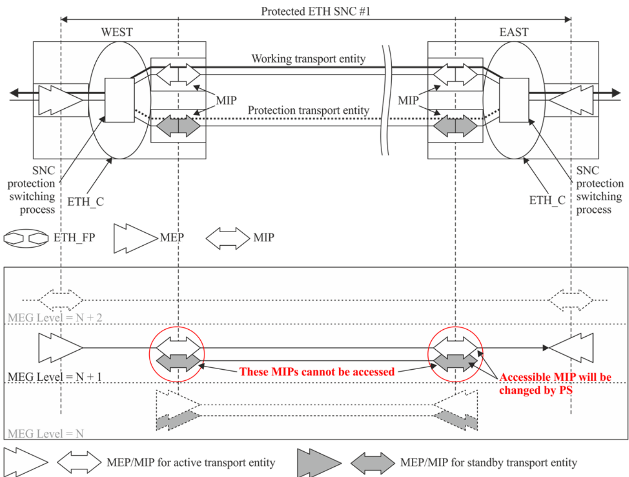
図 III.1/JT-G8031 –双方向プロテクション切替のためのMEPとMIP
