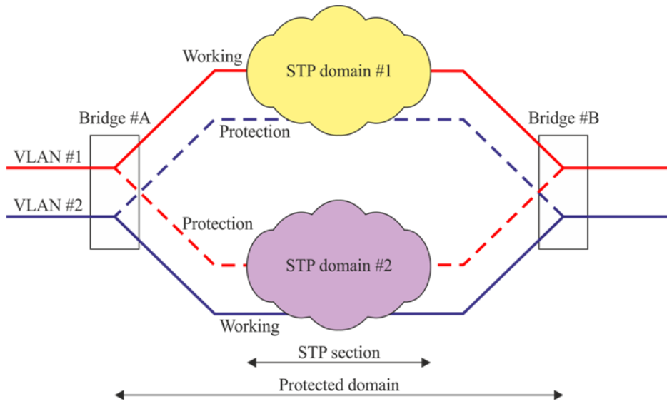
図 II.3/JT-G8031 - VLANごとに保護ドメインとSTPドメイン間で重複が有るケース
