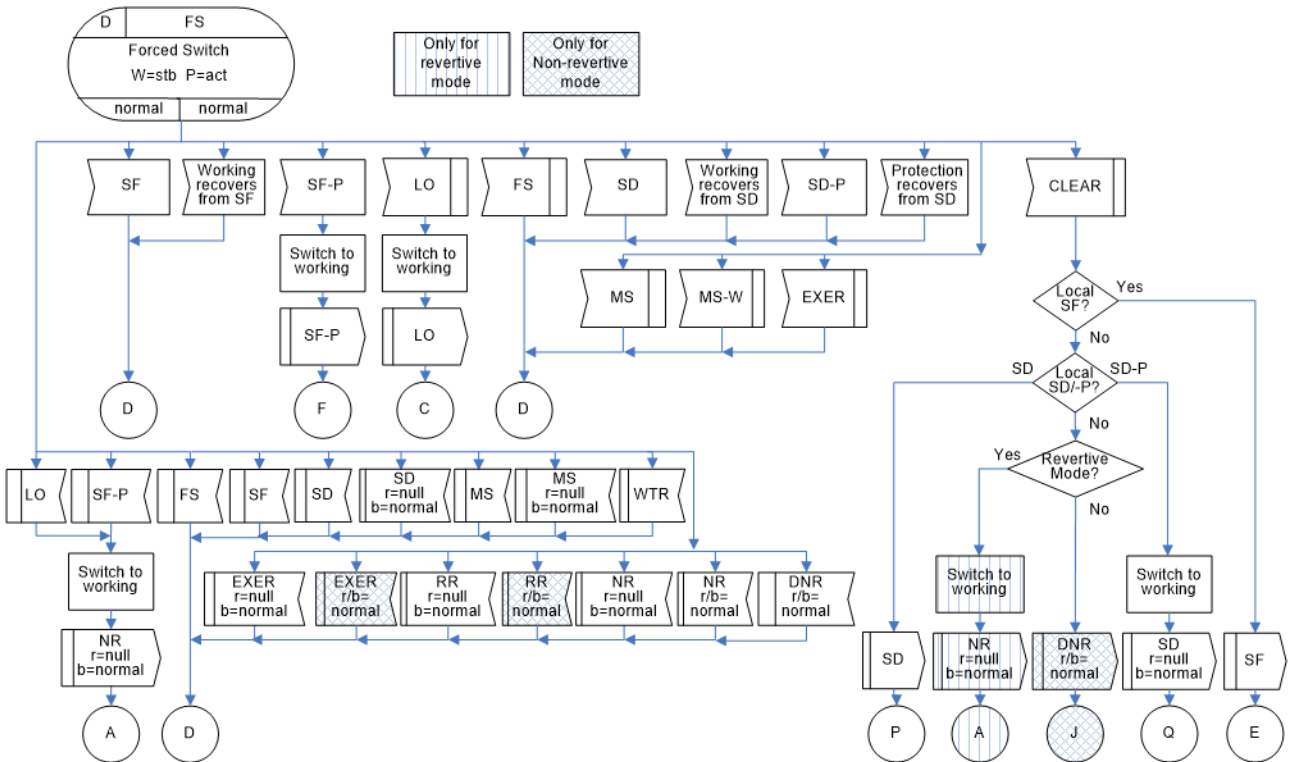
図 IV.20/JT-G8031 - 1+1双方向プロテクション切替におけるFS(r/b=normal)状態
