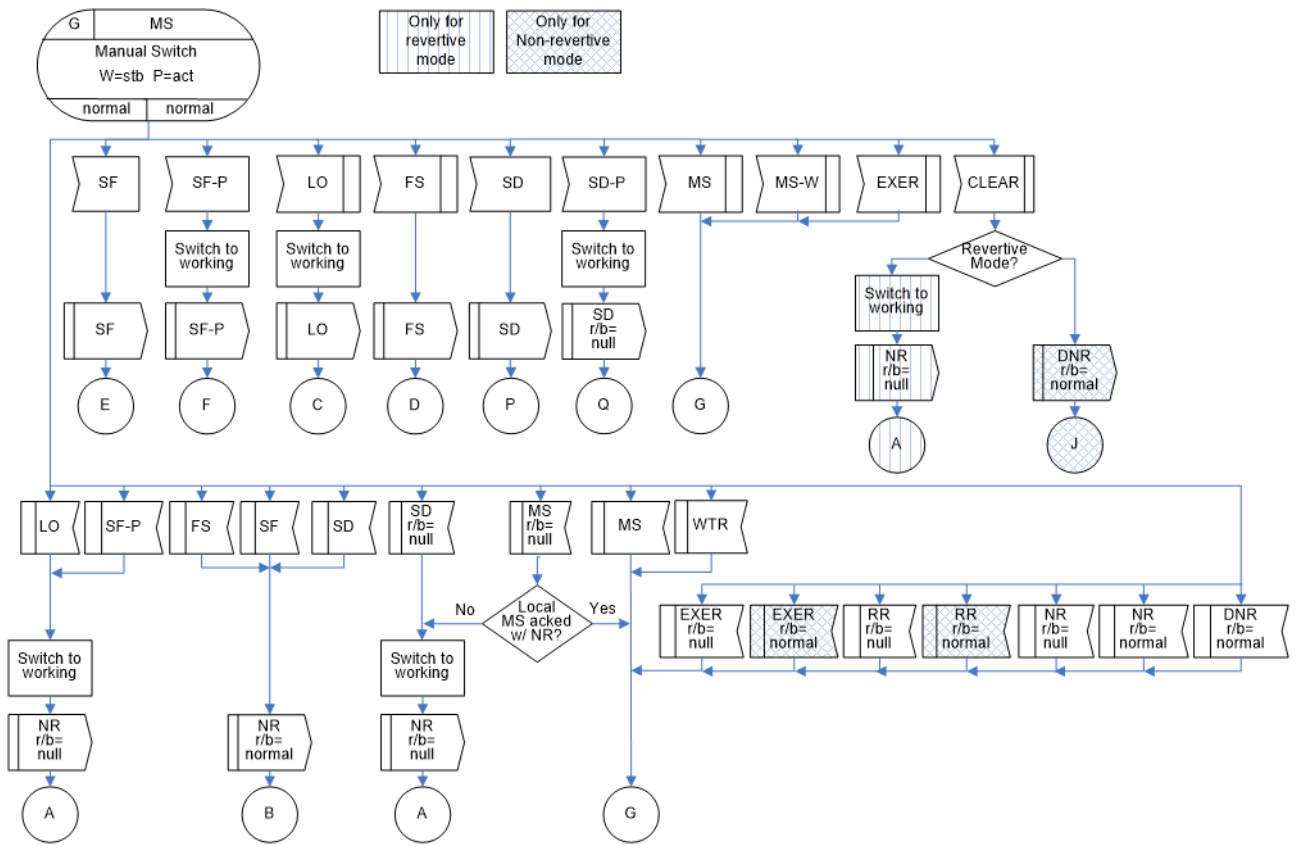
図 IV.7/JT-G8031 -1:1双方向プロテクション切替におけるMS(r/b=normal)状態
