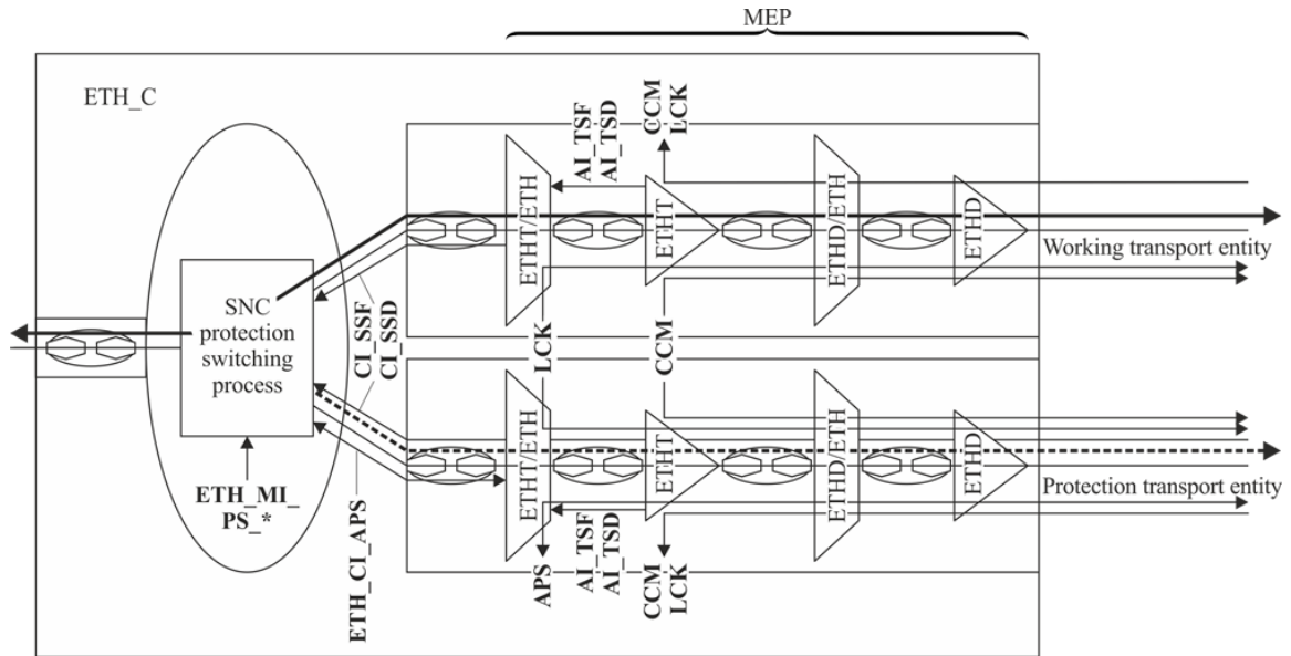
図10-3/ JT-G8031 – プロテクションアーキテクチャにおけるMEPとSNC両方のプロテクション切替の振舞い
