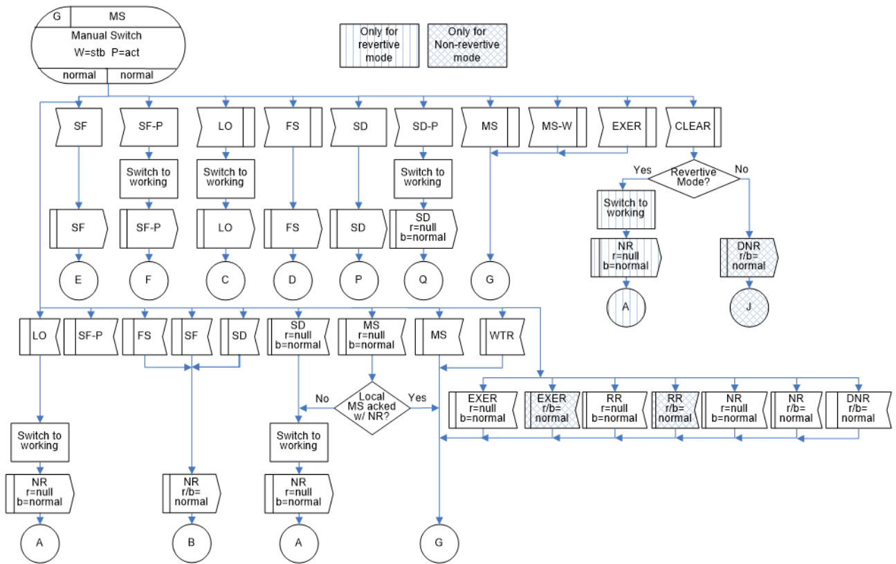
図 IV.23/JT-G8031 - 1+1双方向プロテクション切替におけるMS(r/b=normal)状態
