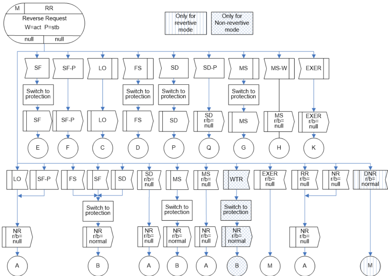
図 IV.13/JT-G8031 - 1:1双方向プロテクション切替におけるRR(r/b=null)状態
