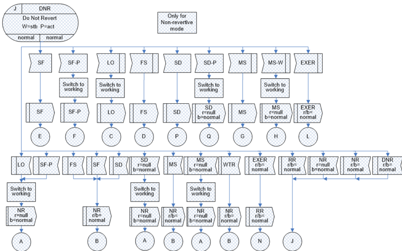
図 IV.26/JT-G8031 - 1+1双方向プロテクション切替におけるDNR(r/b=normal)状態
