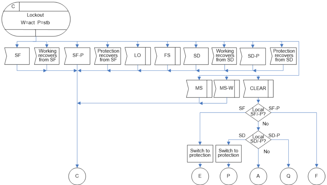
図 IV.34/JT-G8031 - 1+1片方向プロテクション切替におけるLO(W=act / P=stb)状態
