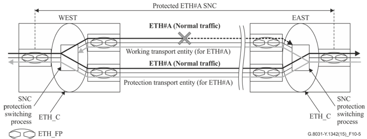
図10-5/ JT-G8031 - 1+1 双方向プロテクションアーキテクチャ -運用系エンティティの信号故障（または信号劣化）状態
