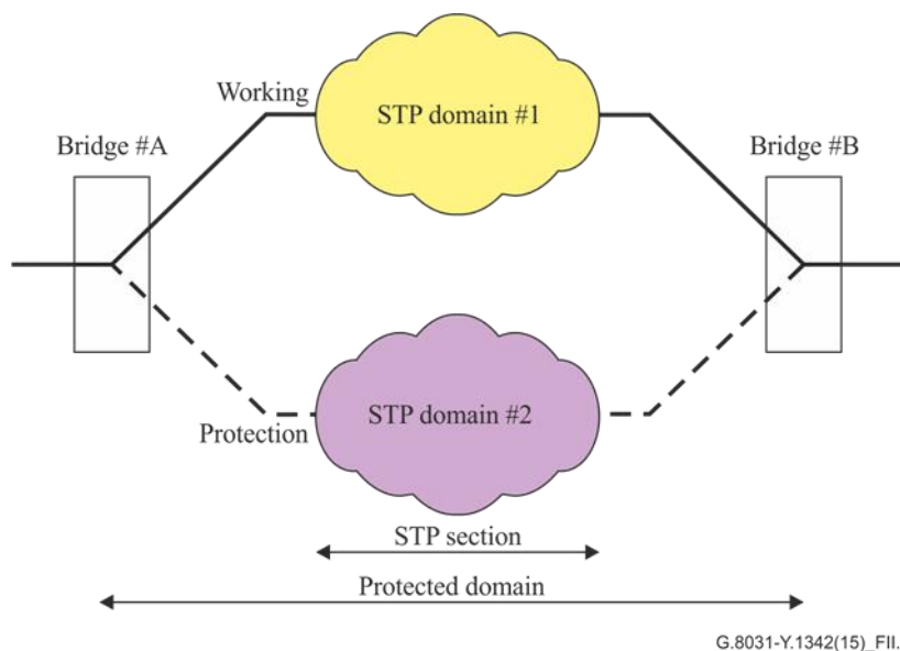
図 II.2/JT-G8031 -保護ドメインとSTPドメイン間で重複が有るケース
