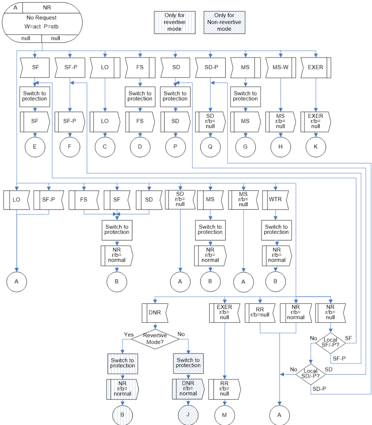
図 IV.1/JT-G8031 - 1:1双方向プロテクション切替におけるNR(r/b=null)状態
