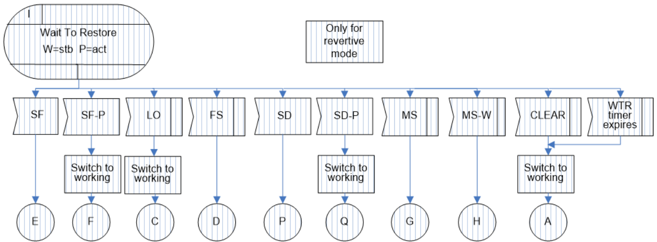
図 IV.40/JT-G8031 -1+1片方向プロテクション切替におけるWTR(W=stb / P=act)状態
