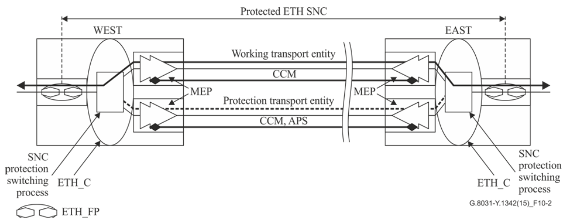
図10-2/ JT-G8031 – プロテクションアーキテクチャにおけるMEPs
