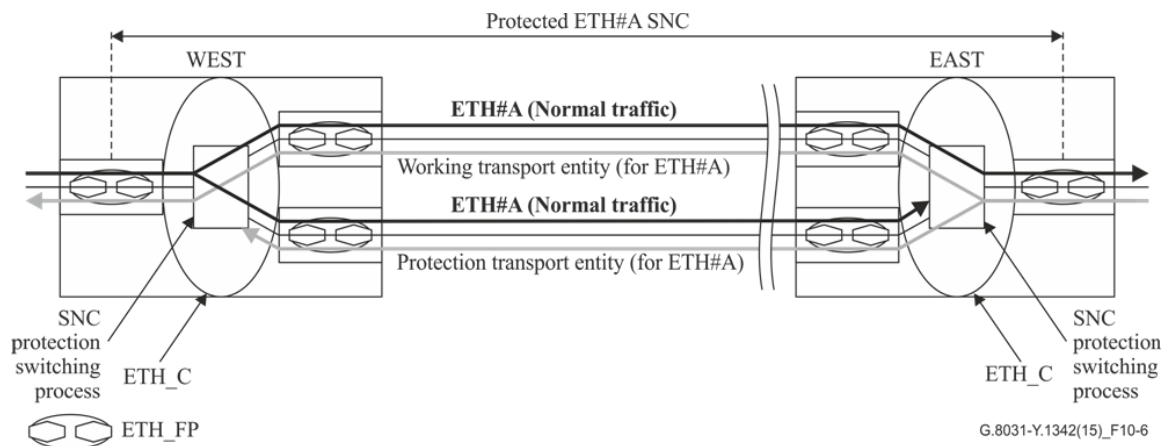
図10-6/ JT-G8031 - 1+1 片方向プロテクションアーキテクチャ
