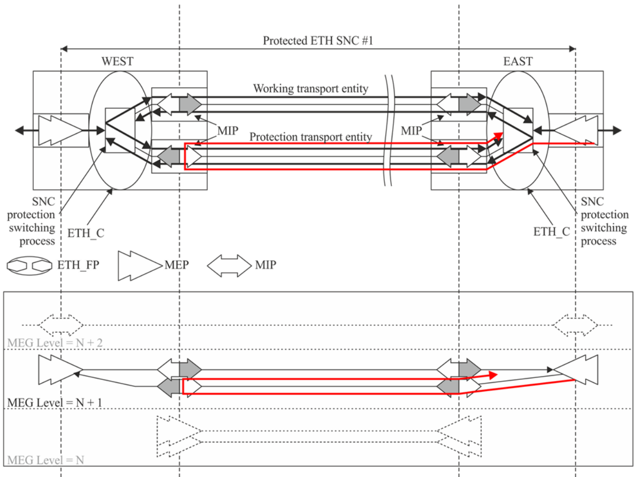
図 III.2/JT-G8031 - 1+1片方向プロテクション切替のためのMEPとMIP
