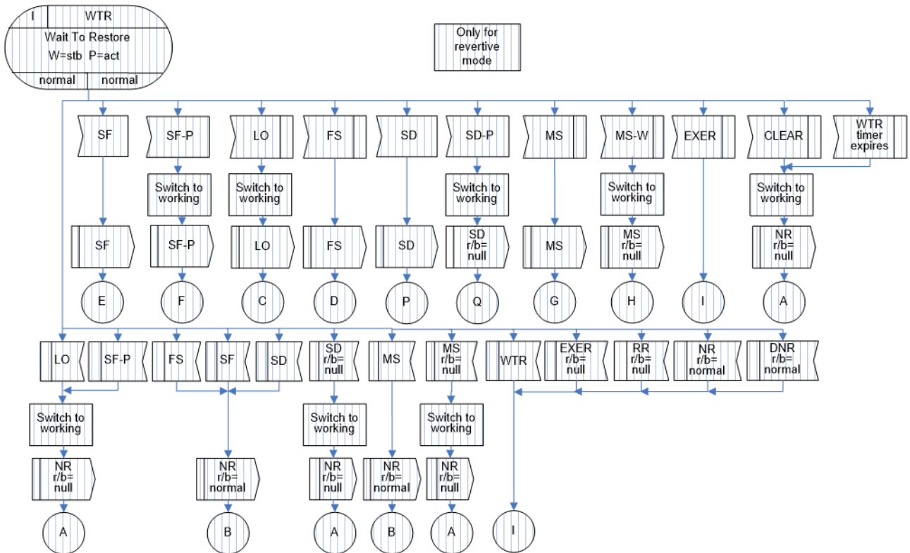
図 IV.9/JT-G8031 - 1:1双方向プロテクション切替におけるWTR(r/b=normal)状態
