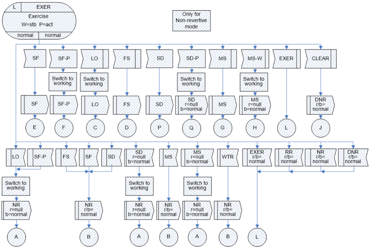
図 IV.28/JT-G8031 - 1+1双方向プロテクション切替におけるEXER(r/b=normal)状態
