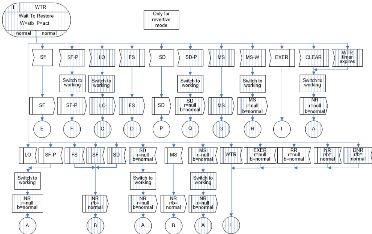
図 IV.25/JT-G8031 - 1+1双方向プロテクション切替におけるWTR(r/b=normal)状態
