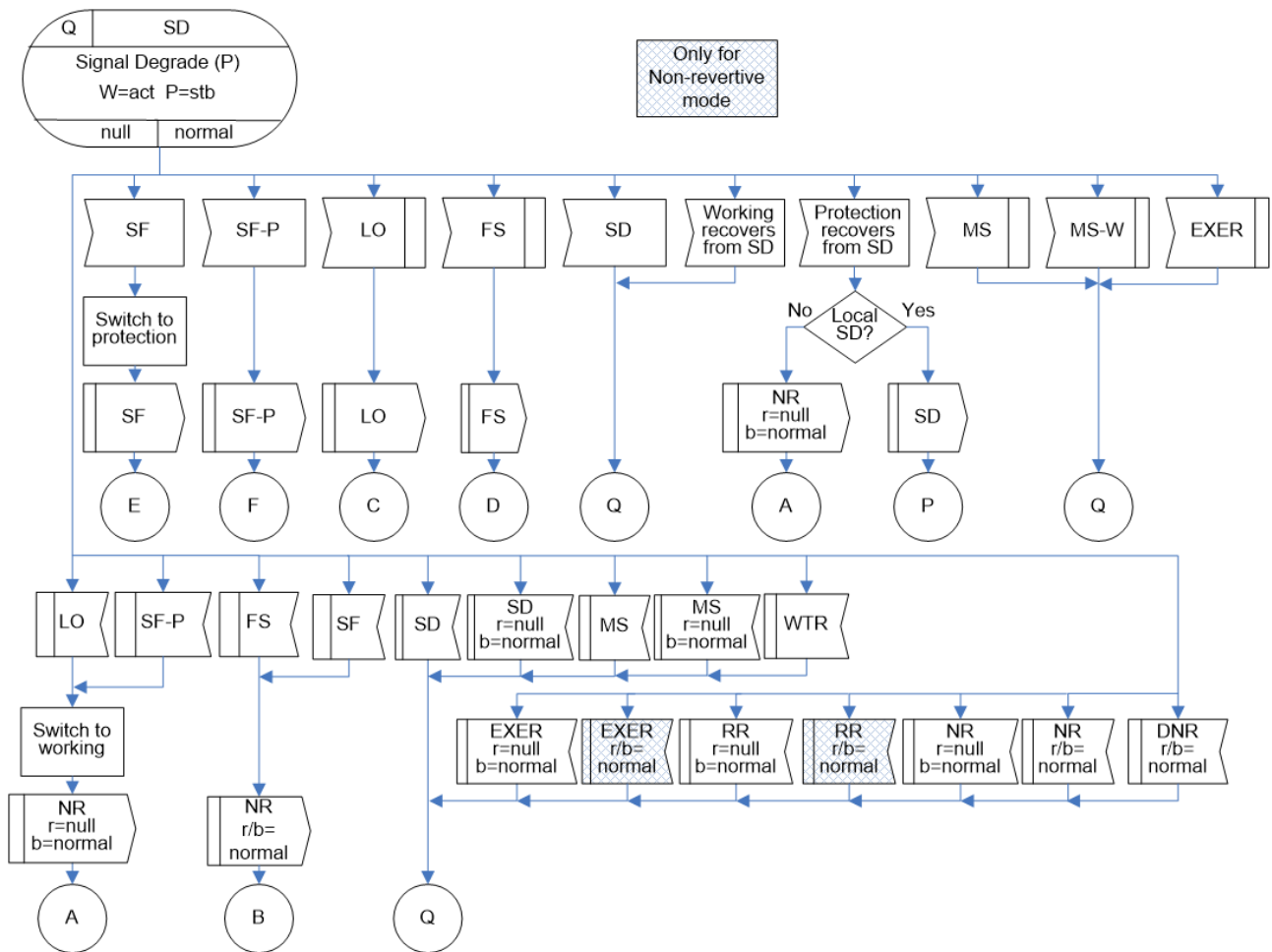
図 IV.32/JT-G8031 - 1+1双方向プロテクション切替におけるSD(r=null, b=normal)状態
