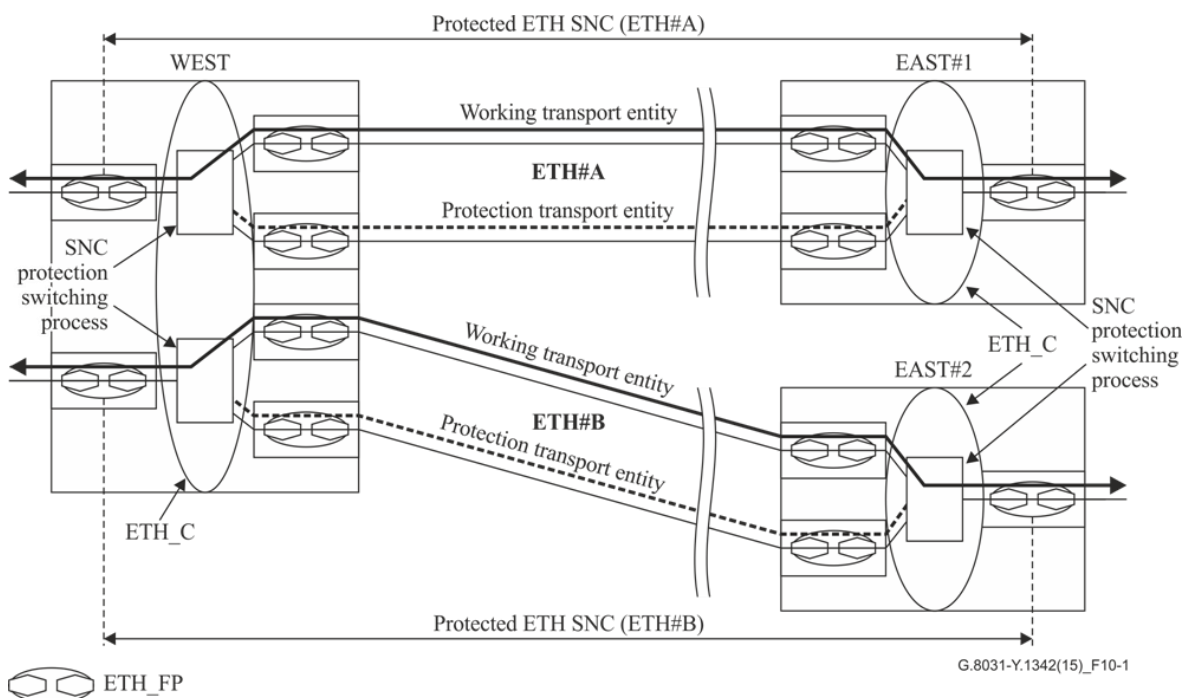
図 10-1/JT-G8031 – ETH SNC/S プロテクションアーキテクチャ
