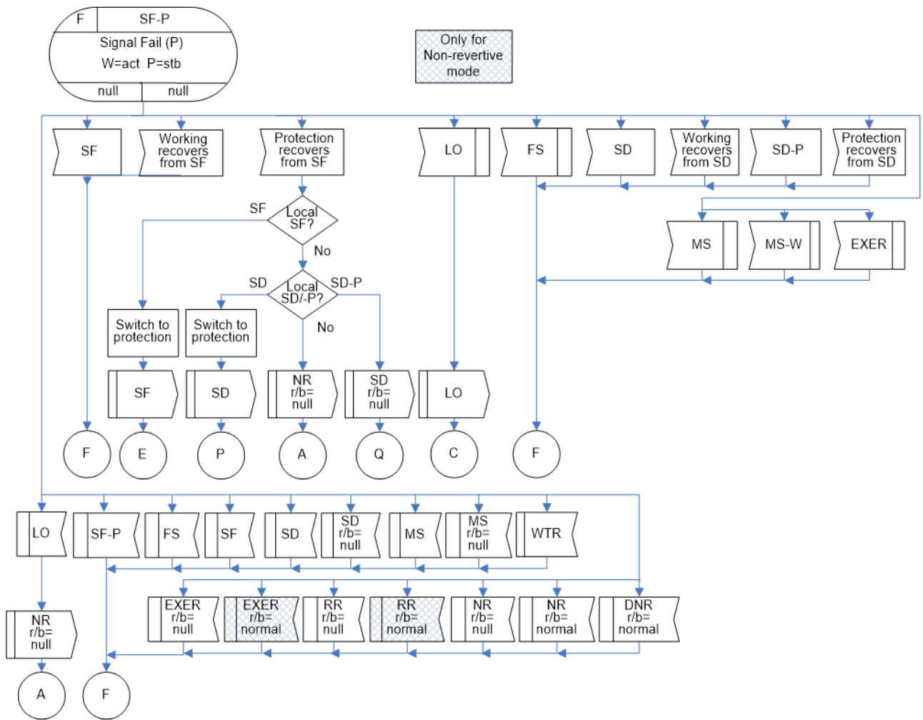
図 IV.6/JT-G8031 - 1:1双方向プロテクション切替におけるSF-P(r/b=null)状態
