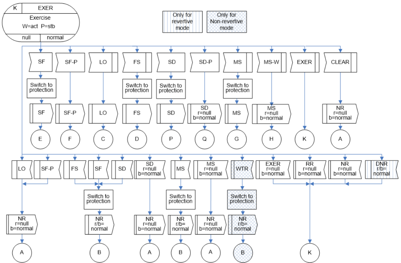
図 IV.27/JT-G8031 - 1+1双方向プロテクション切替におけるEXER(r=null, b=normal)状態
