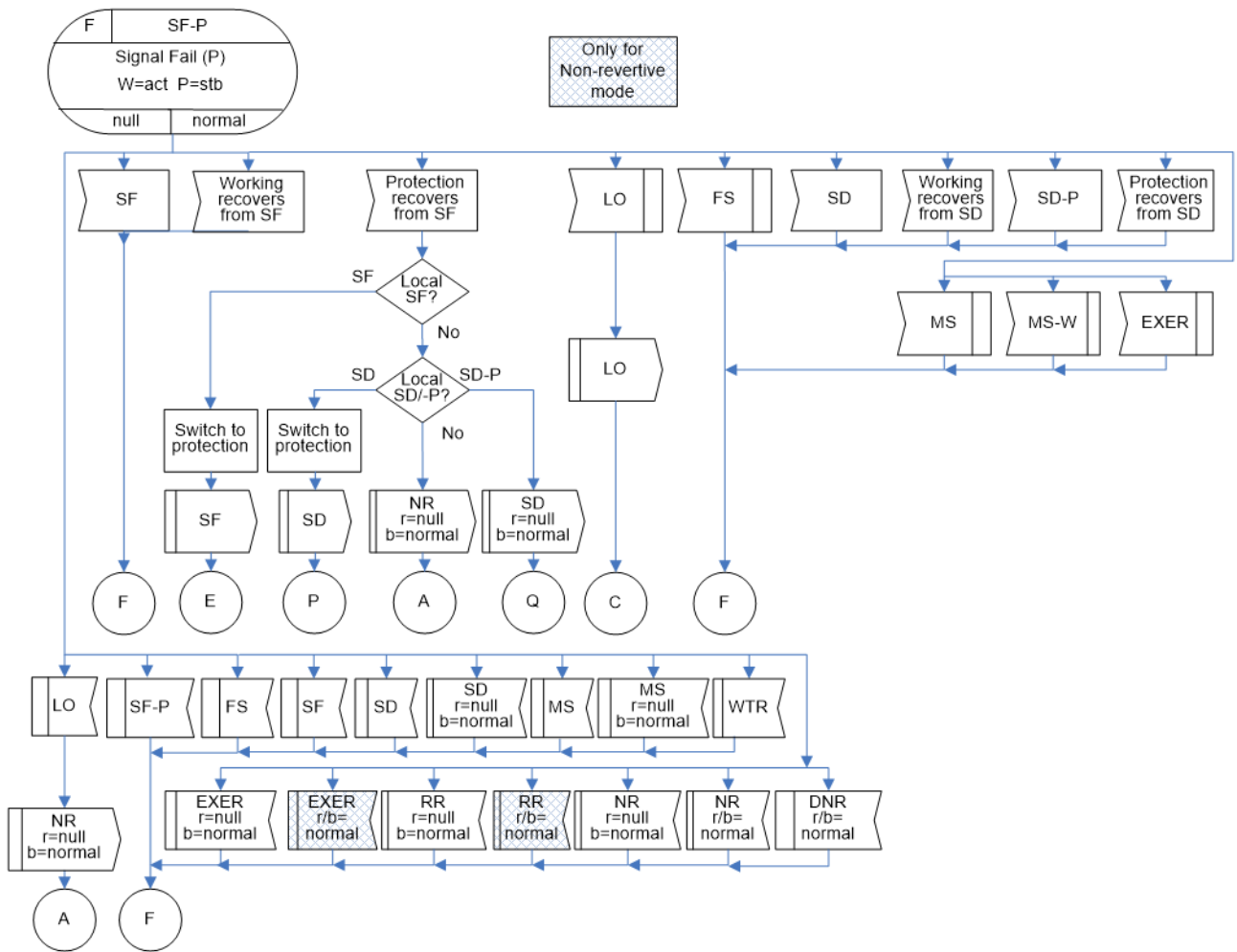
図 IV.22/JT-G8031 - 1+1双方向プロテクション切替におけるSF-P( r=null, b=normal )状態
