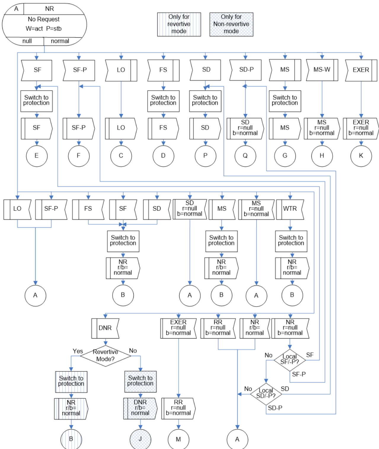
図 IV.17/JT-G8031 - 1+1双方向プロテクション切替におけるNR(r=null, b=normal)状態
