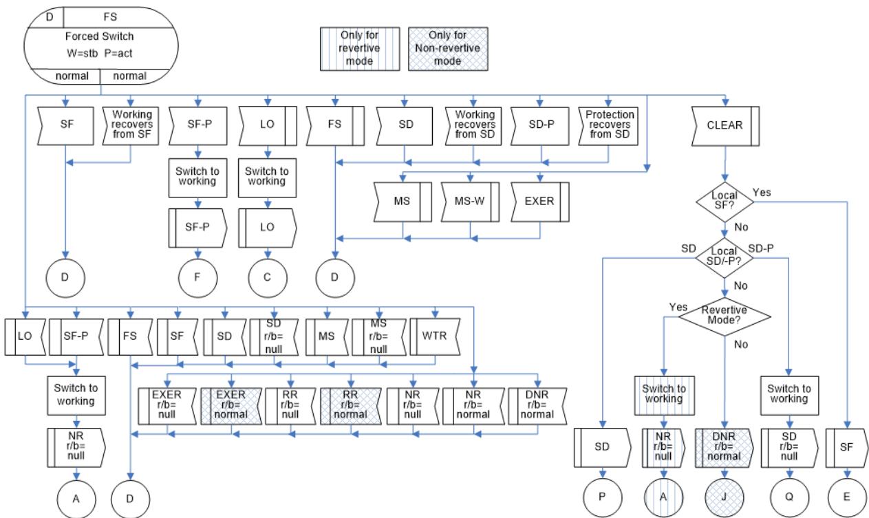
図 IV.4/JT-G8031 - 1:1双方向プロテクション切替におけるFS(r/b=normal)状態
