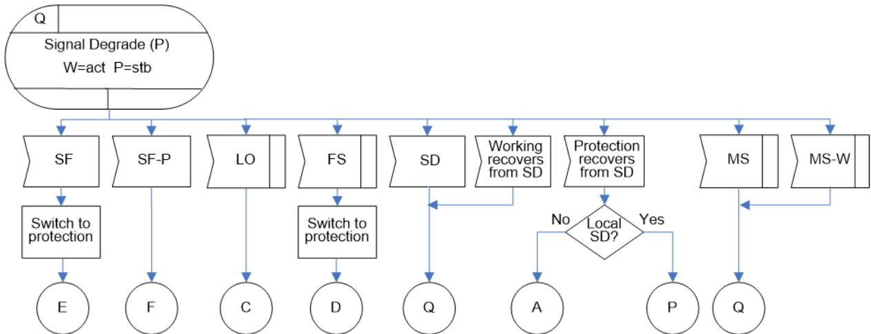
図 IV.43/JT-G8031 - 1+1片方向プロテクション切替におけるSD(W=act / P=stb)状態
