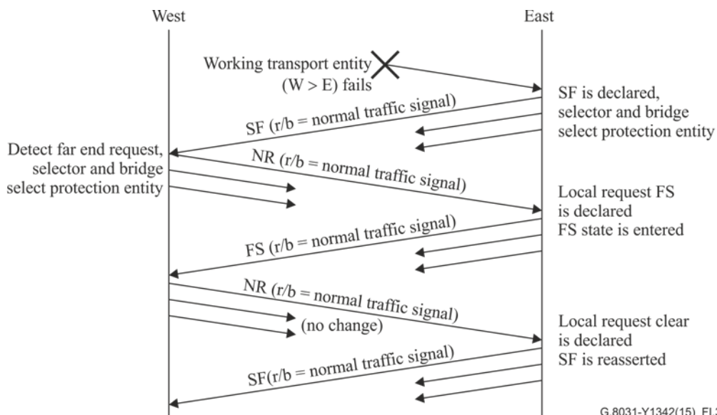
図 I.2/JT-G8031 - プロトコル例(非切り戻しモード)
