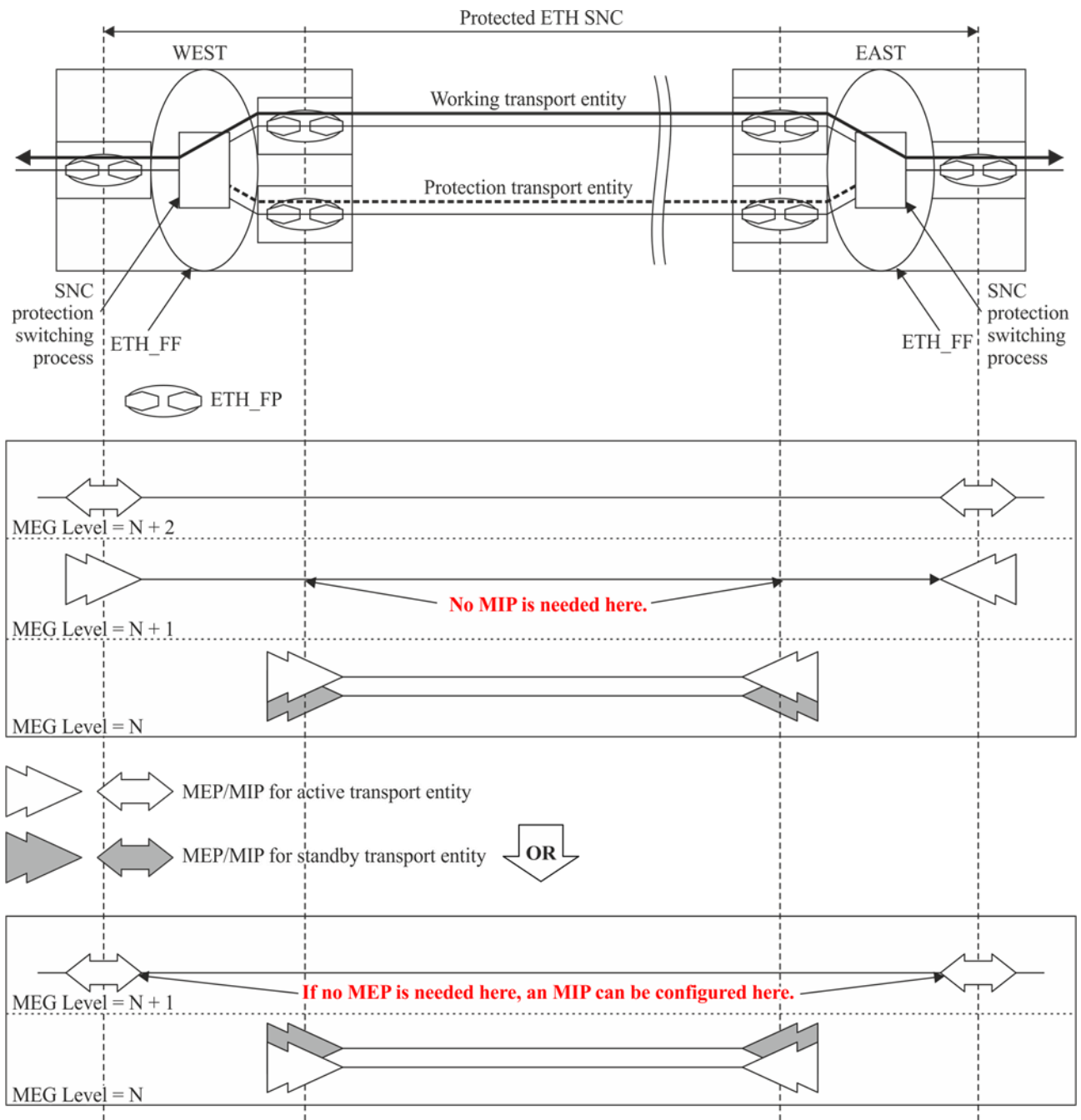
図 III.3/JT-G8031 -プロテクション切替環境のためのMEPとMIPの構成例
