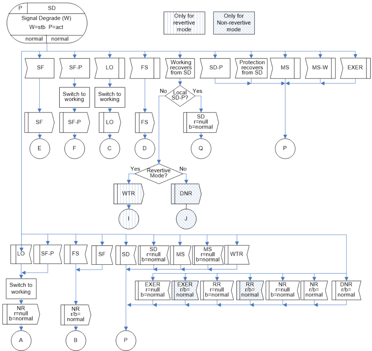
図 IV.31/JT-G8031 - 1+1双方向プロテクション切替におけるSD(r/b=normal)状態
