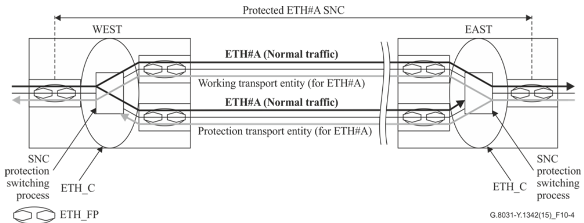
図10-4/ JT-G8031 –1+1 双方向プロテクションアーキテクチャ
