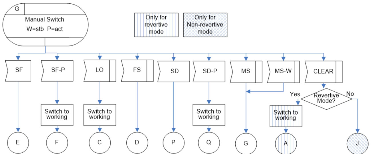
図 IV.38/JT-G8031 -1+1片方向プロテクション切替におけるMS(W=stb / P=act)状態
