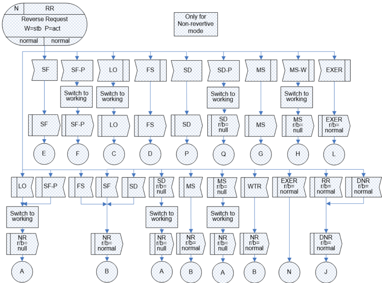
図 IV.14/JT-G8031 - 1:1双方向プロテクション切替におけるRR(r/b=normal)状態
