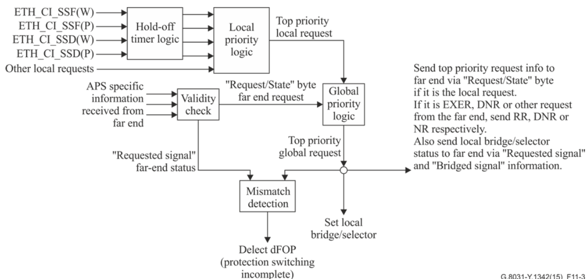
図11-3/JT-G8031 -1+1/1:1 リニアプロテクション切替アルゴリズムの原則
