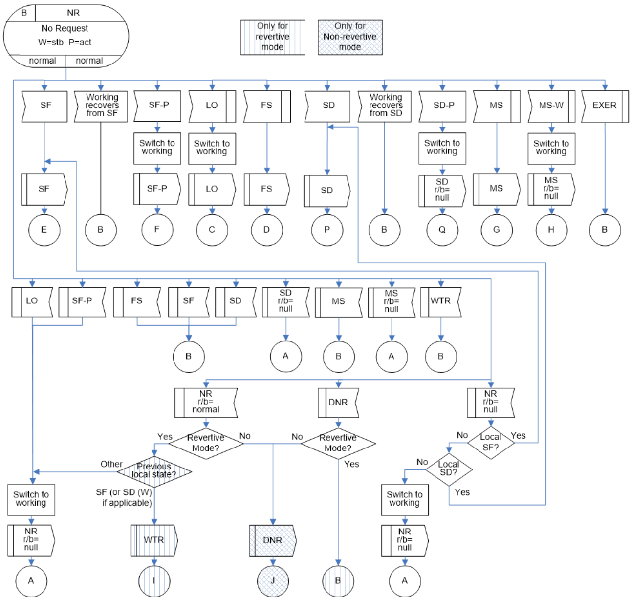
図 IV.2/JT-G8031 - 1:1双方向プロテクション切替におけるNR(r/b=normal)状態
