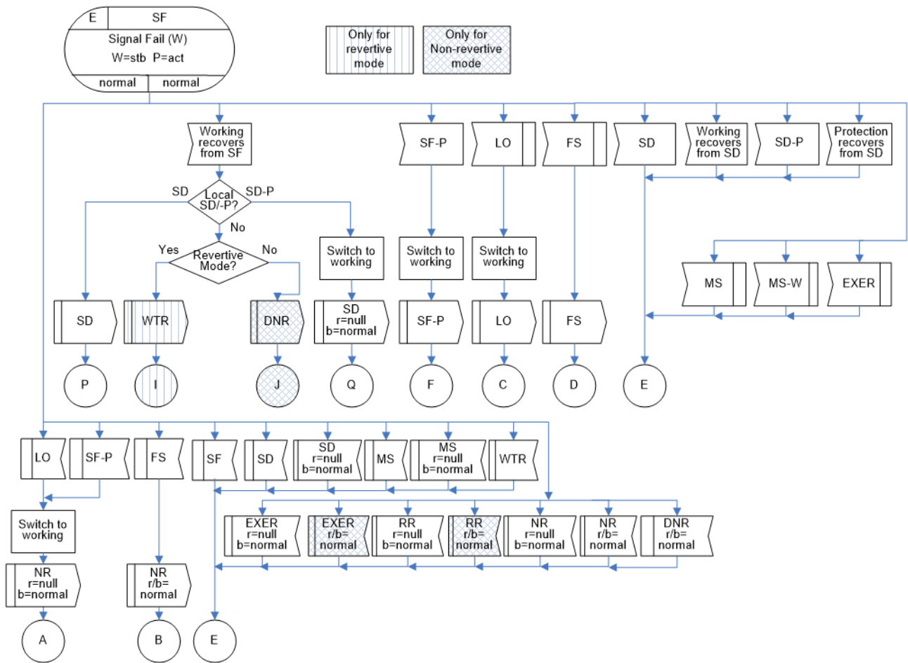
図 IV.21/JT-G8031 - 1+1双方向プロテクション切替におけるSF(r/b=normal)状態
