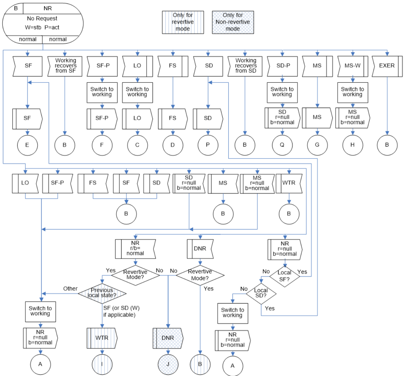
図 IV.18/JT-G8031 - 1+1双方向プロテクション切替におけるNR(r/b=normal)状態
