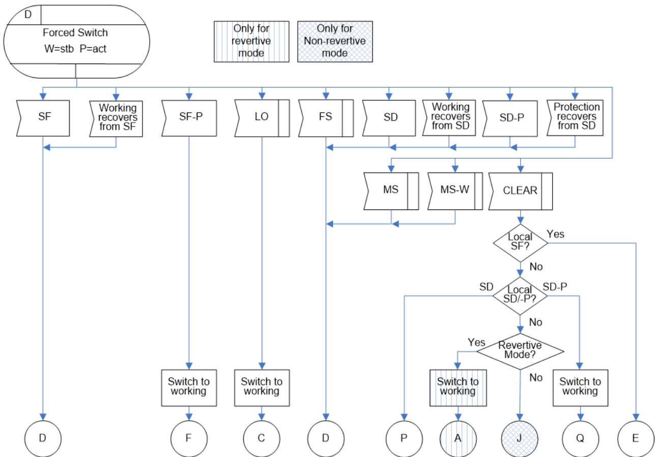
図 IV.35/JT-G8031 - 1+1片方向プロテクション切替におけるFS(W=stb / P=act)状態
