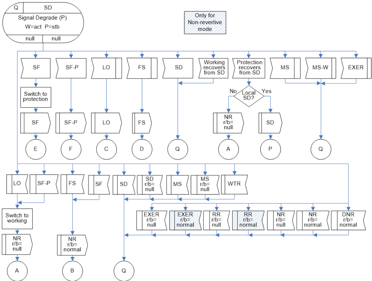
図 IV.14/JT-G8031 – 1:1 双方向プロテクション切替におけるSD(r/b=null)状態
