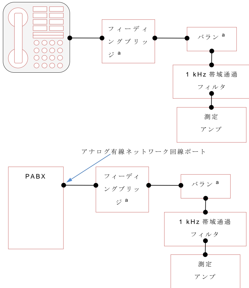
図 G.7- アナログ有線ネットワーク回線の復調測定するための試験構成例
