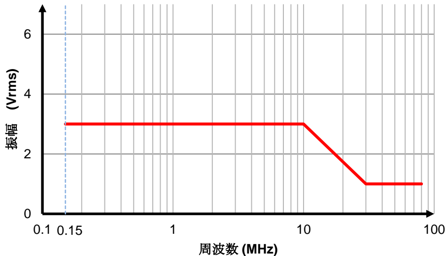
図 3 – 表の項 2.1 に定義されている連続性誘導 RF 妨害波レベルのグラフ表示 (10)
