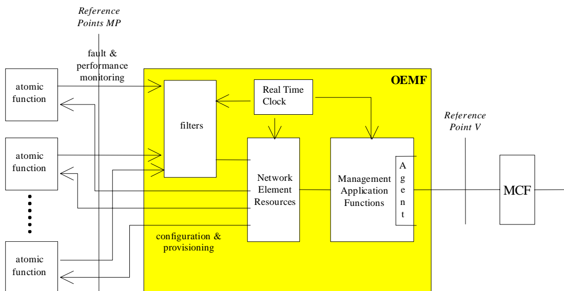
Figure 7/G.874: 光要素管理機能(OEMF)
