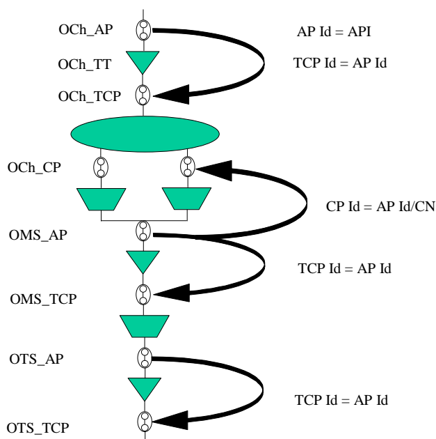
図 7/G.874: CP と TCP 識別子スキーマ
