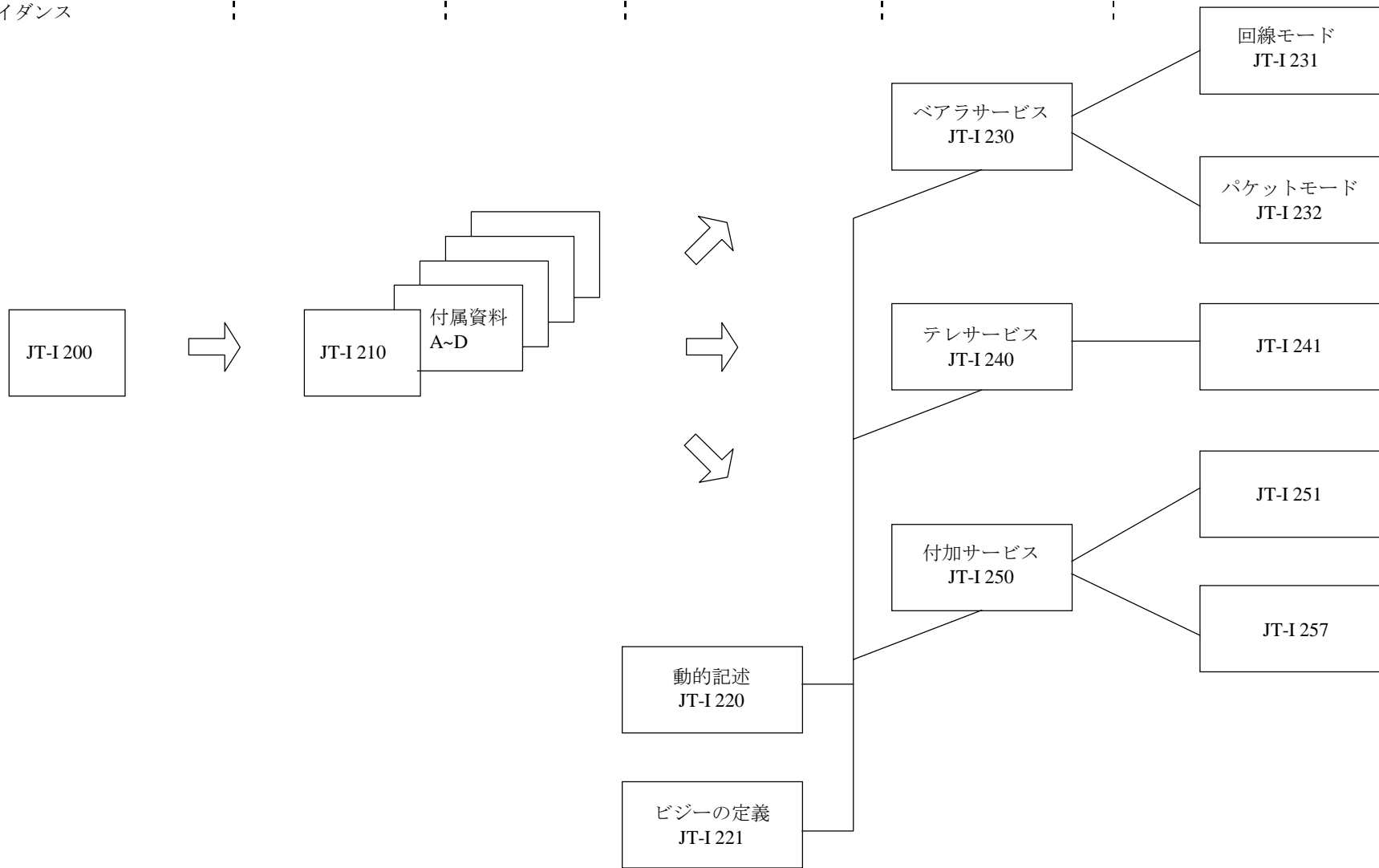
図 2-1 / JT-I 200 (CCITT I.200) 標準 JT-I 200シリーズの構造
