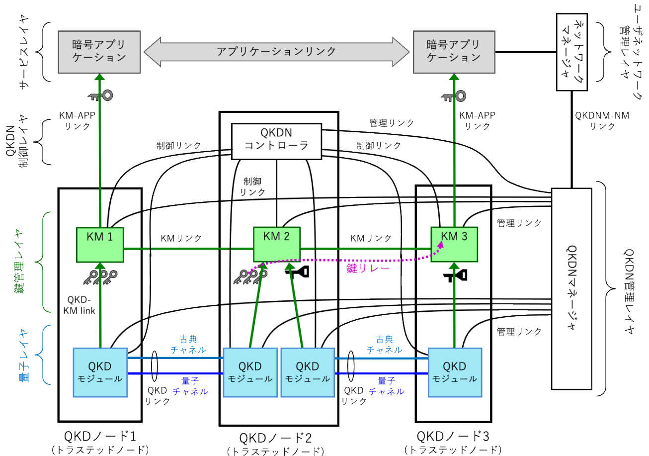
図2 QKDNとユーザネットワークの典型的な構成
