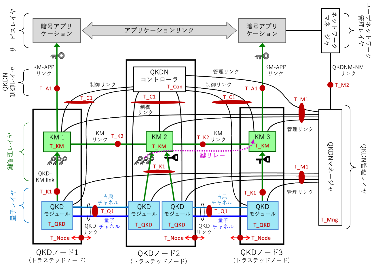
図3 QKDNのセキュリティ脅威
